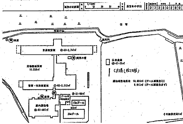
(配置図)
