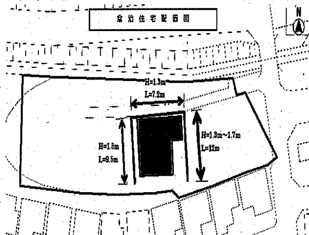
(配置図)
