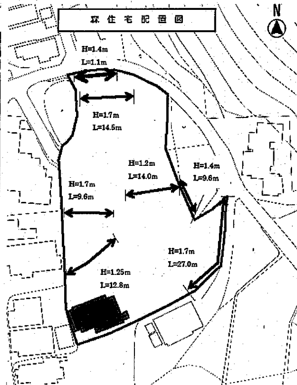
(配置図)
