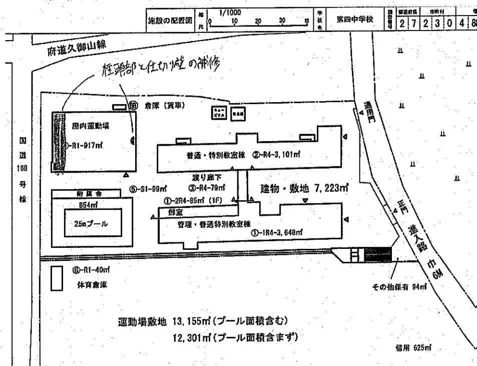
No.15 (配置図)
