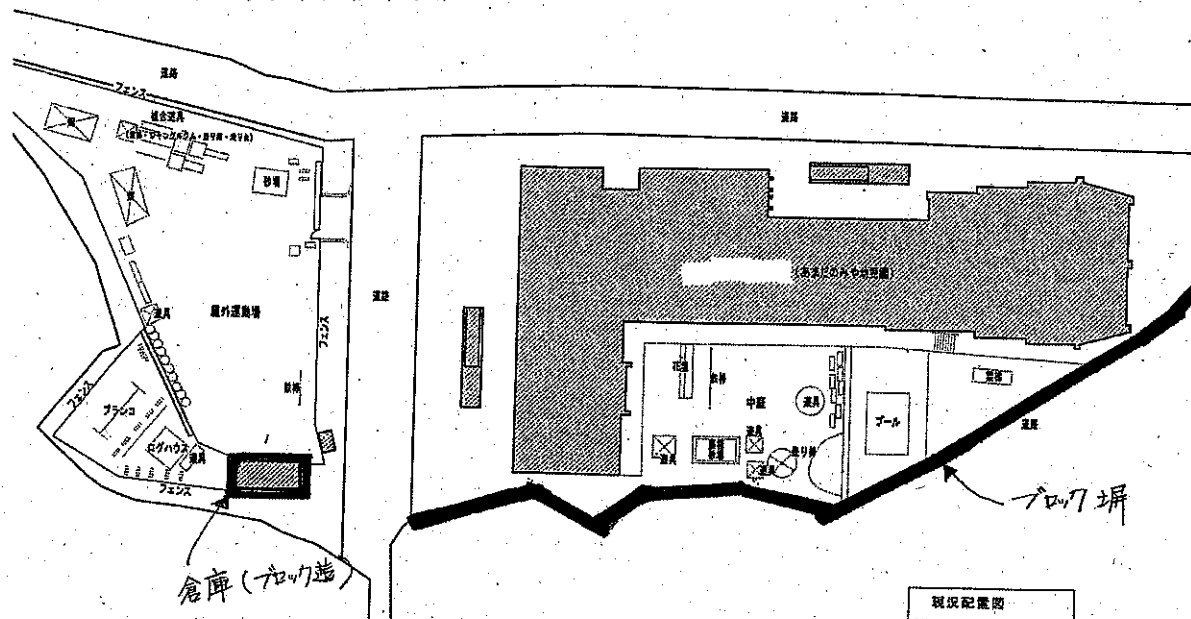
No.19 あまだのみや幼稚園 (配置図)
